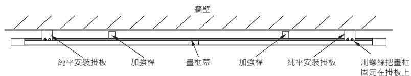
圖21 純平面畫框幕掛板安裝示意圖(頂視圖)
