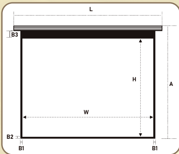
正視圖
