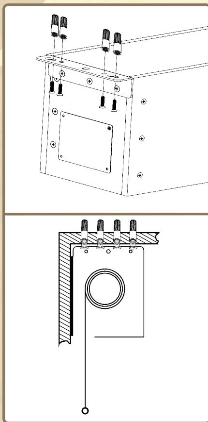
頂裝式
