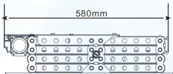
側視圖
